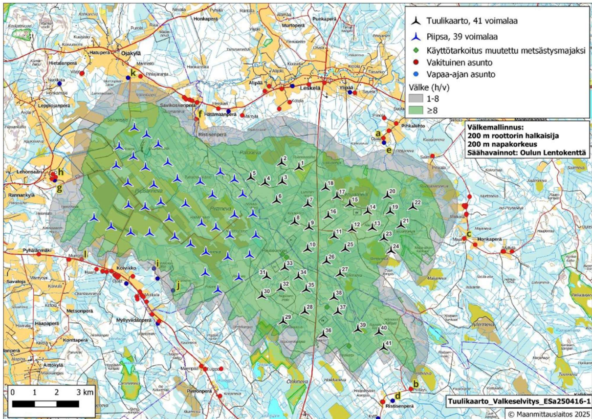
Kuva 76. Tuulikaarron kaavien neljän kaava-alueen sekä Piipsannevan tuulivoimapauston yhteisvaikutuksen välkemallinnus.
