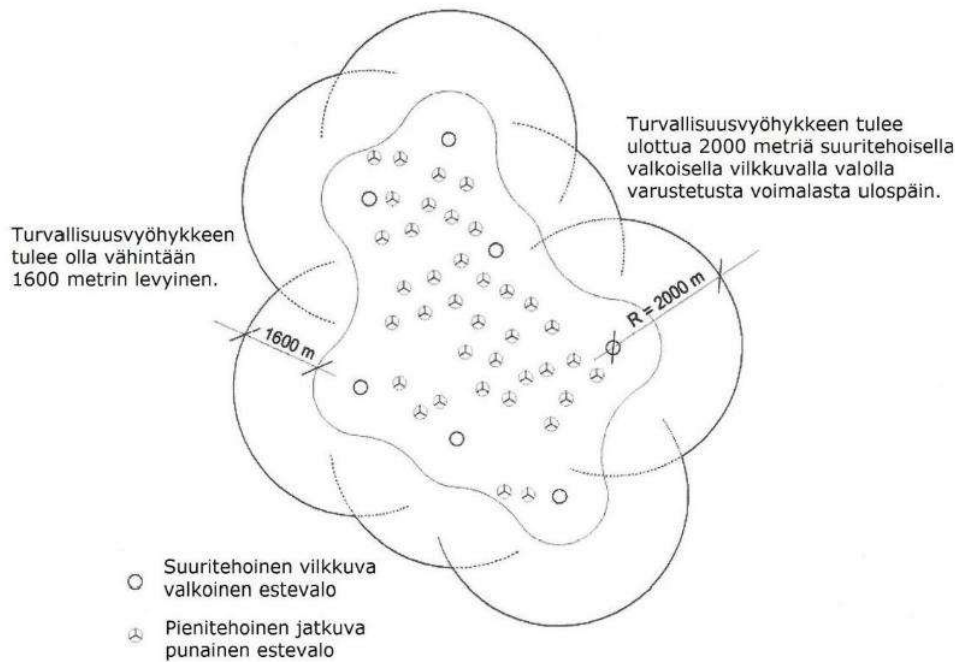
Kuva 80. Lentoestevalojen sijoitteluesimerkki, kun tuulivoimapaiston voimaloiden korkein pyyhkäisykohta on yli 150 metriä maanpinnasta. Tuulivoimaloiden ulkokehän muodostavat suuritehoiset B-tyypin vilkkuvat valkoiset lentoestevalot. (Traficom 2020)
