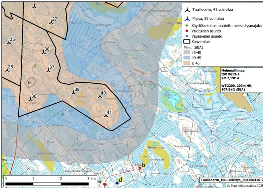
Kuva 75. Yhteisvaikutusten melumallinnus. Kärsämäki itäinen kaava-alue.
