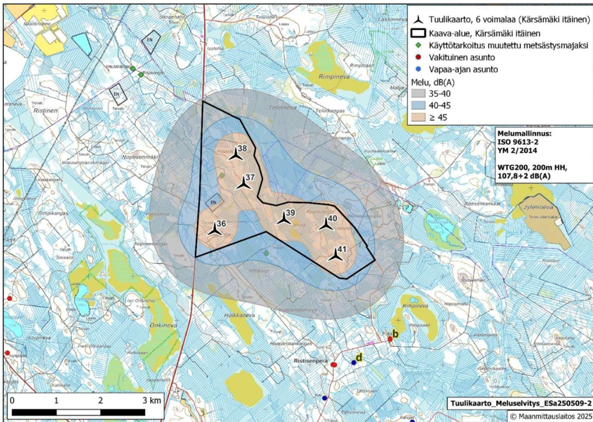
Kuva 50. Kärsämäki itä -osayleiskaavan tuulivoimaloiden melumallinnus.
