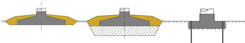
Kuva 81. Tuulivoimalat voidaan perustaa useilla eri tavoilla. Periaatekuvat maanvaraisesta teräsbetoniperustuk-sesta, teräsbetoniperustuksesta massanvaihdon kanssa sekä kallioankkuroidusta teräsbetoniperustuksesta.
