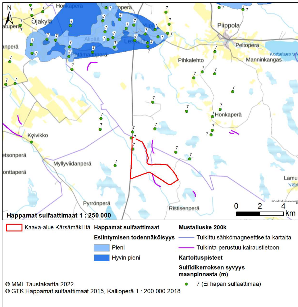
Kuva 34. Happamien sulfaattimaiden esiintymispotentiaali hankealueen läheisyydessä (Lähde: GTK).
