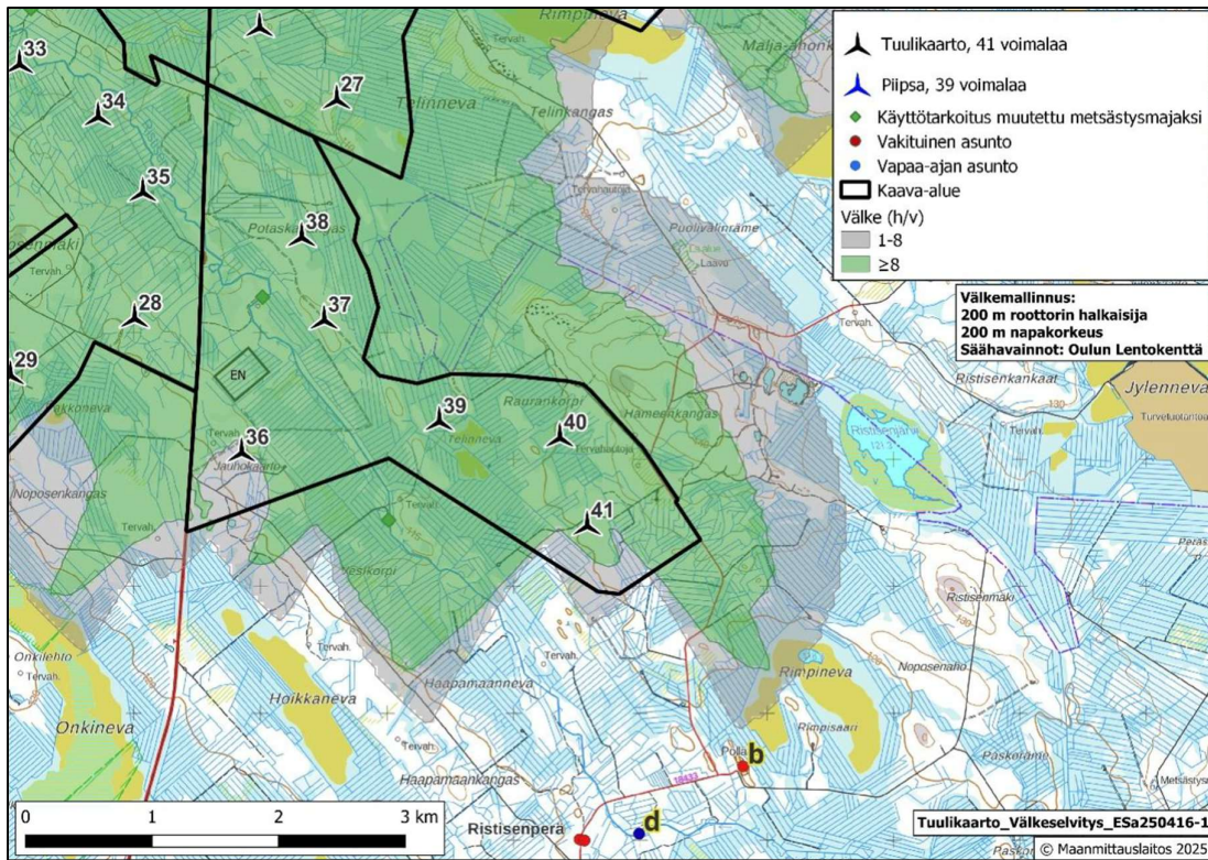
Kuva 77. Varjovälkkeen muodostuminen, Kärsämäki itä kaava-alue.
