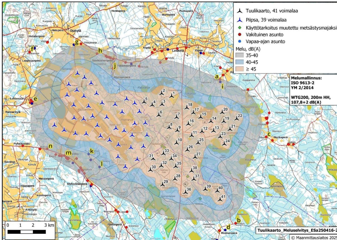
Kuva 74. Melumallinnus yhdessä Piipsannevan voimaloiden kanssa.
