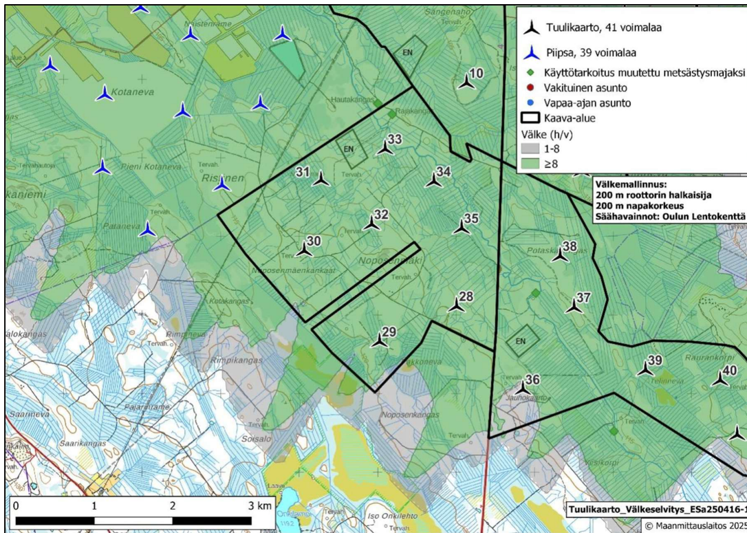
Kuva 79. Varjovälkkeen muodostuminen, Kärsämäki länsi kaava-alue.
