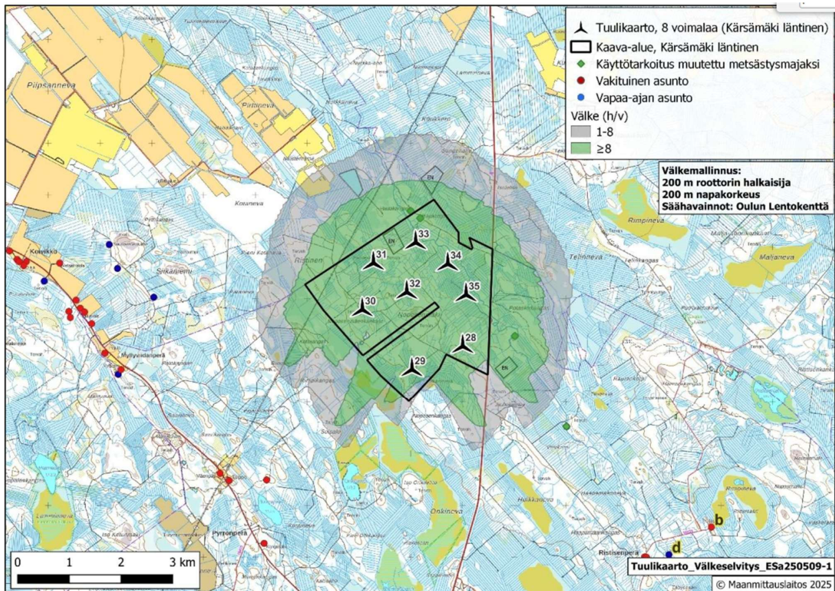
Kuva 53. Valkemallinnuksen tulos Kärsämäki länsi -osayleiskaavan alueella.
