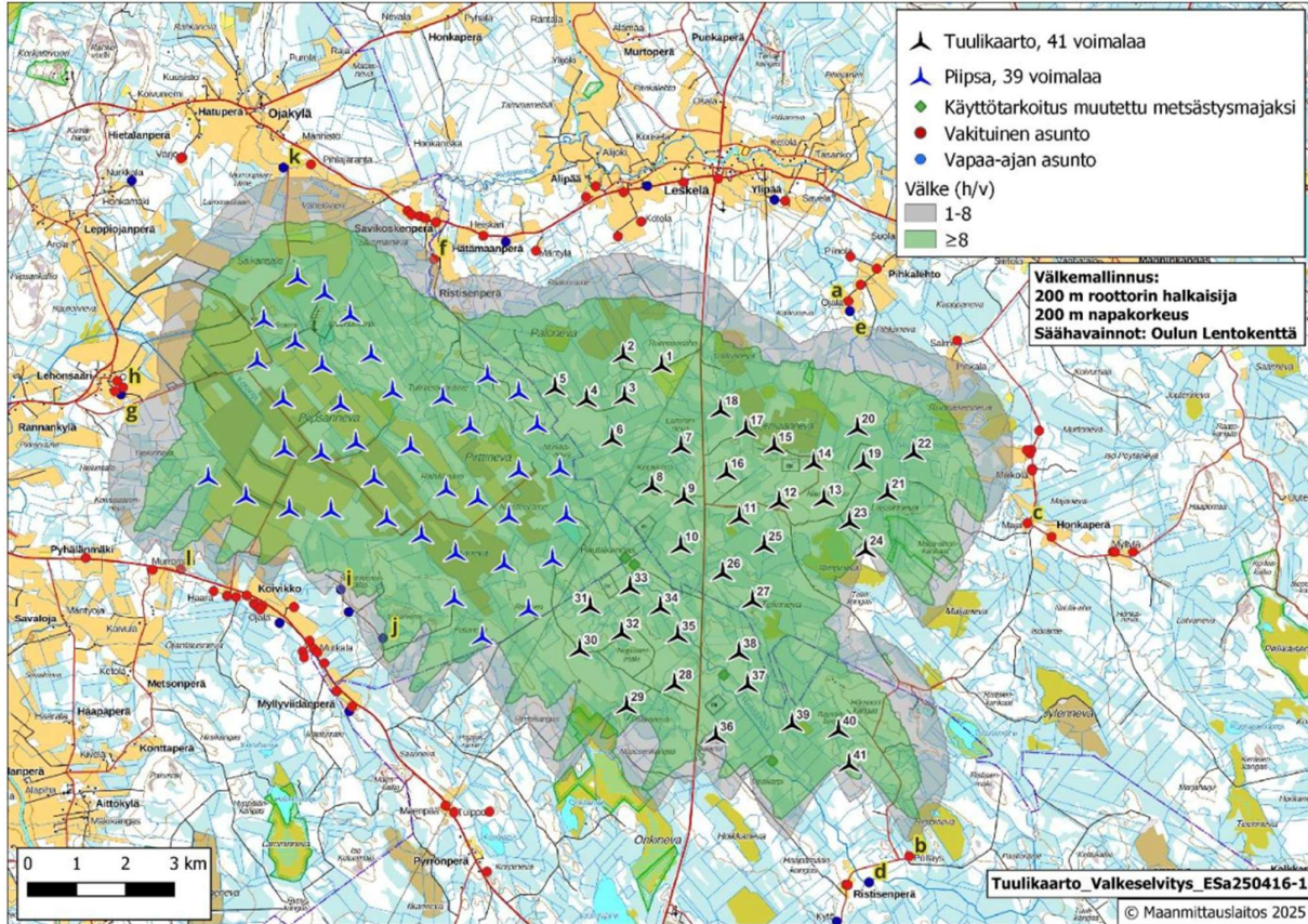
Kuva 78. Tuulikaarron kaikkien neljän kaava-alueen sekä Piipsannevan tuulivoimapuiston yhteisvaikutuksen välkemallinnus.
