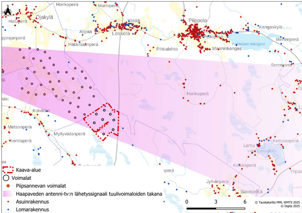
Kuva 65. Haapaveden antenni-tv:n lähetyssignaali Piipsannevan ja Kärsämäki länsi -kaavan voimaloiden takana.
