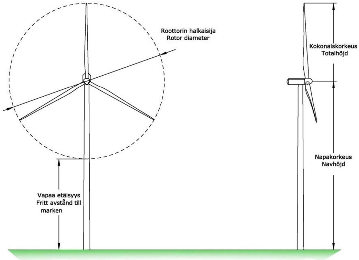
Kuva 80. Tuulivoimalan mallikuva.
