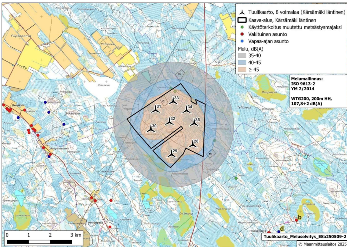
Kuva 52. Kärsämäki länsi-osayleiskaavan tuulivoimaloiden melumallinnus.
