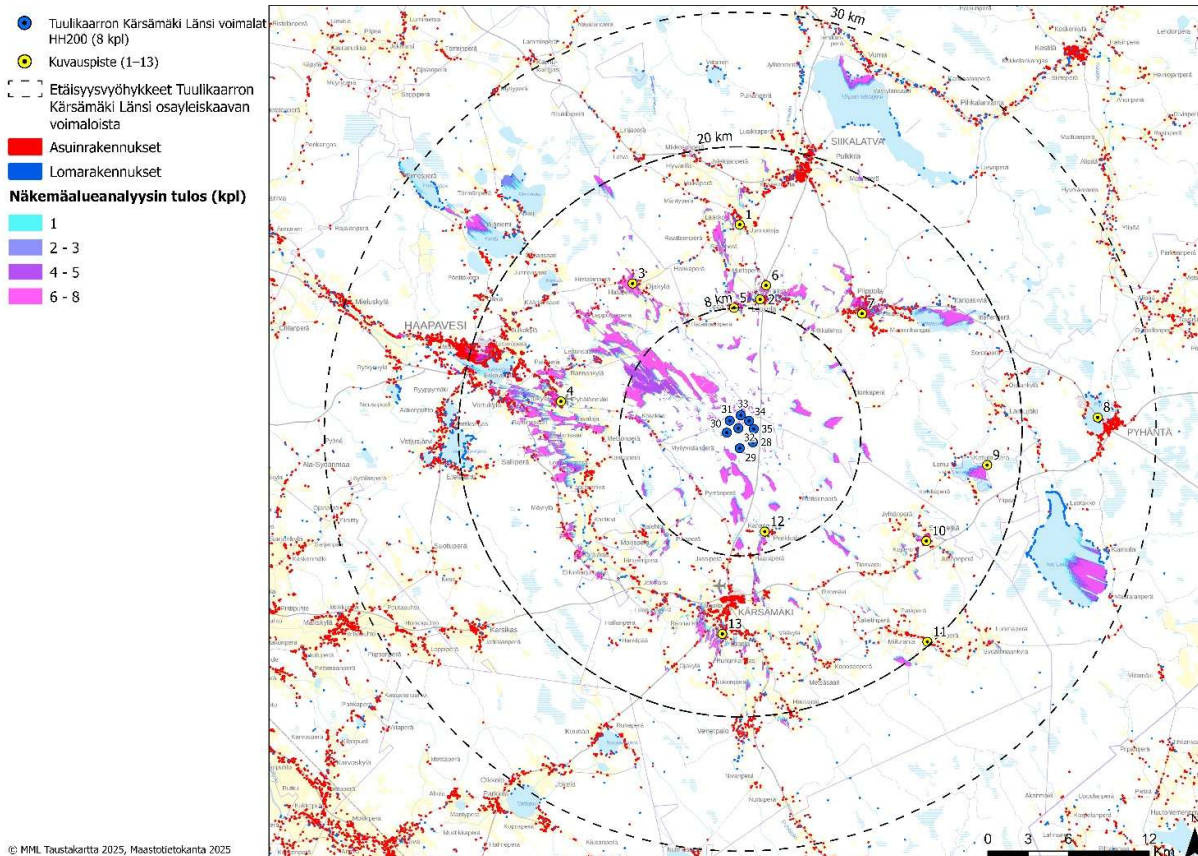
Kuva 15. Näkymäalueanalyysi ja havainnekuva-alueet kartalla.
