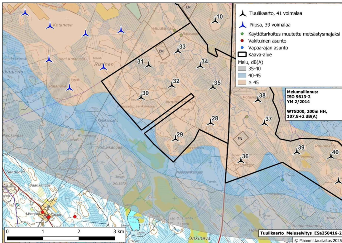
Kuva 77. Yhteisvaikutusten melumallinnus. Kärsämäki läntinen kaava-alue.
