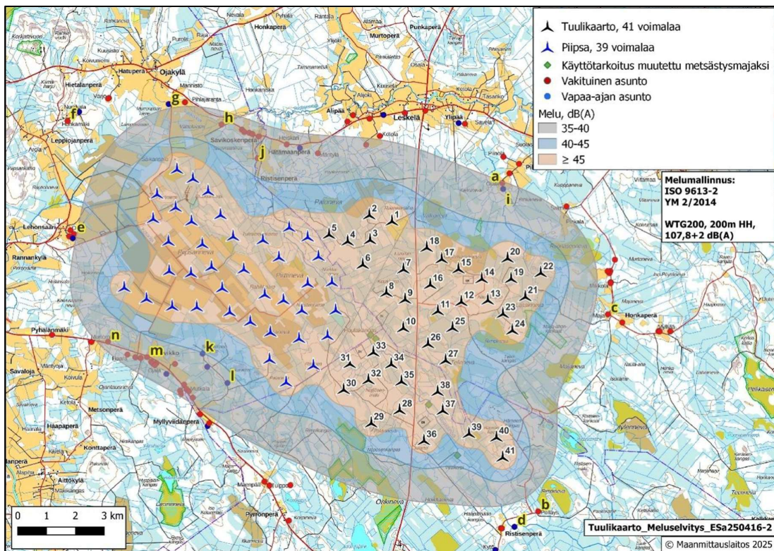
Kuva 76. Melumallinnus yhdessä Piipsannevan voimaloiden kanssa.
