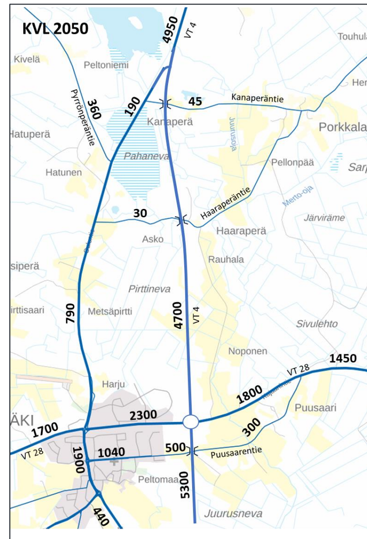
Kuva 12. Ennusteliikennemäärät (KVL, ajon./vrk) yleiskaava-alueen tieverkolla v. 2050.
