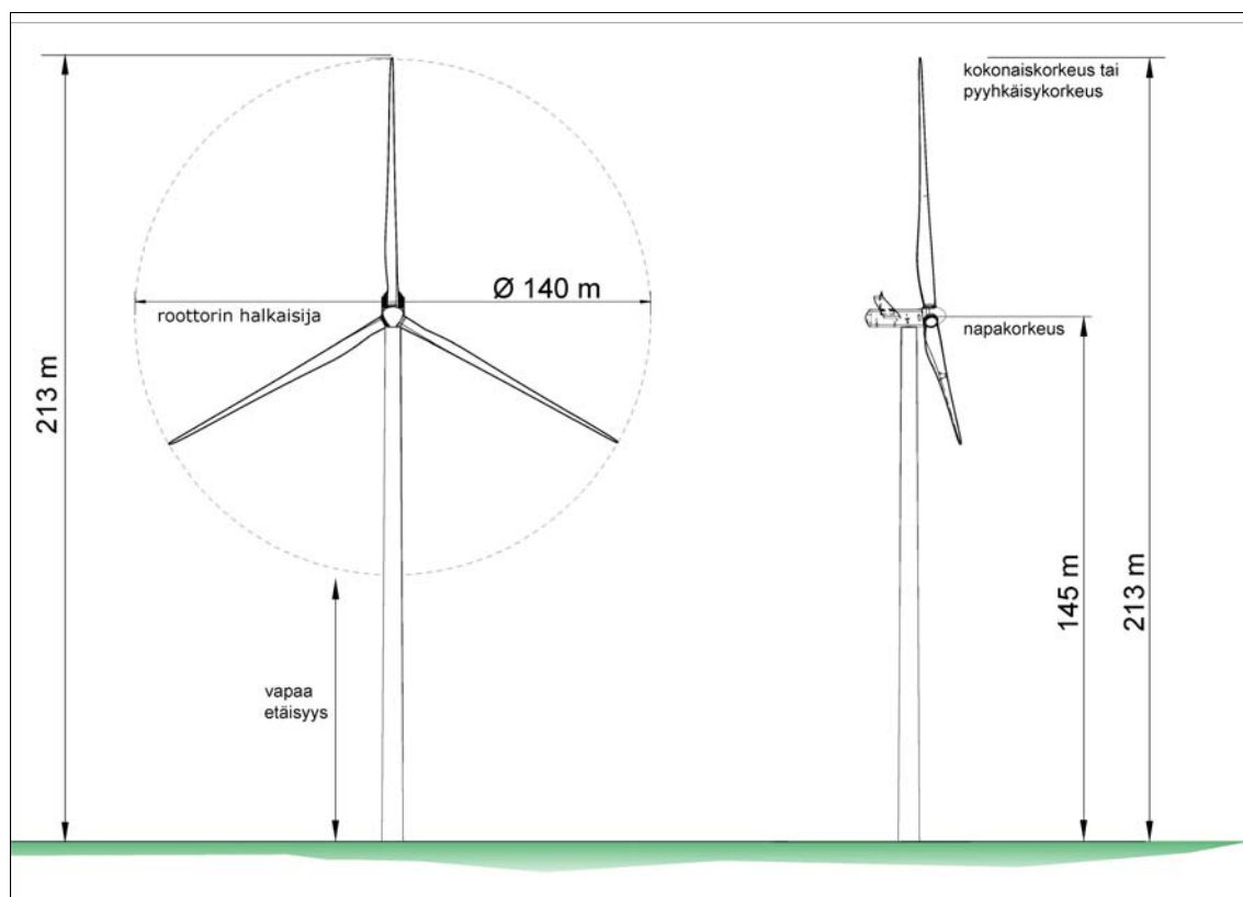
Kuva 19. Mallikuva voimalakorkeudesta.
