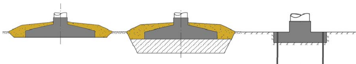
Kuva 20. Tuulivoimalat voidaan perustaa useilla eri tavoilla. Periaatekuvat maanvaraisesta teräsbetoniperustuksesta, teräsbetoniperustuksesta massanvaiholla sekä kallioankkuroidusta teräsbetoniperustuksesta.
